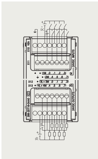
EM DT16
