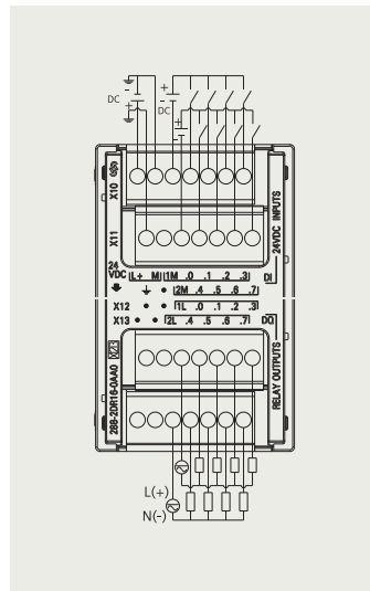
EM DR16
