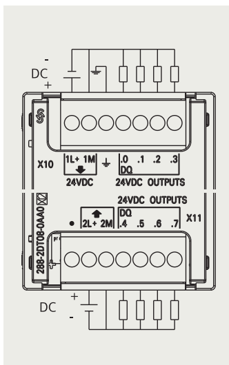
EM DT08
