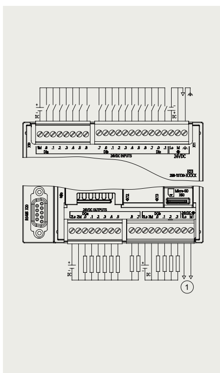
CPU ST30
