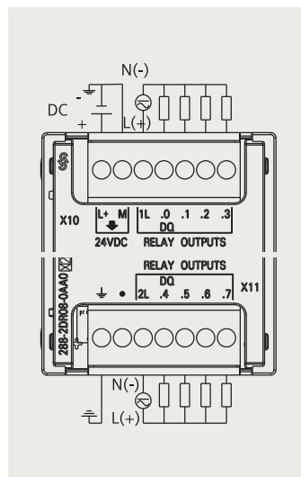
EM DR08
